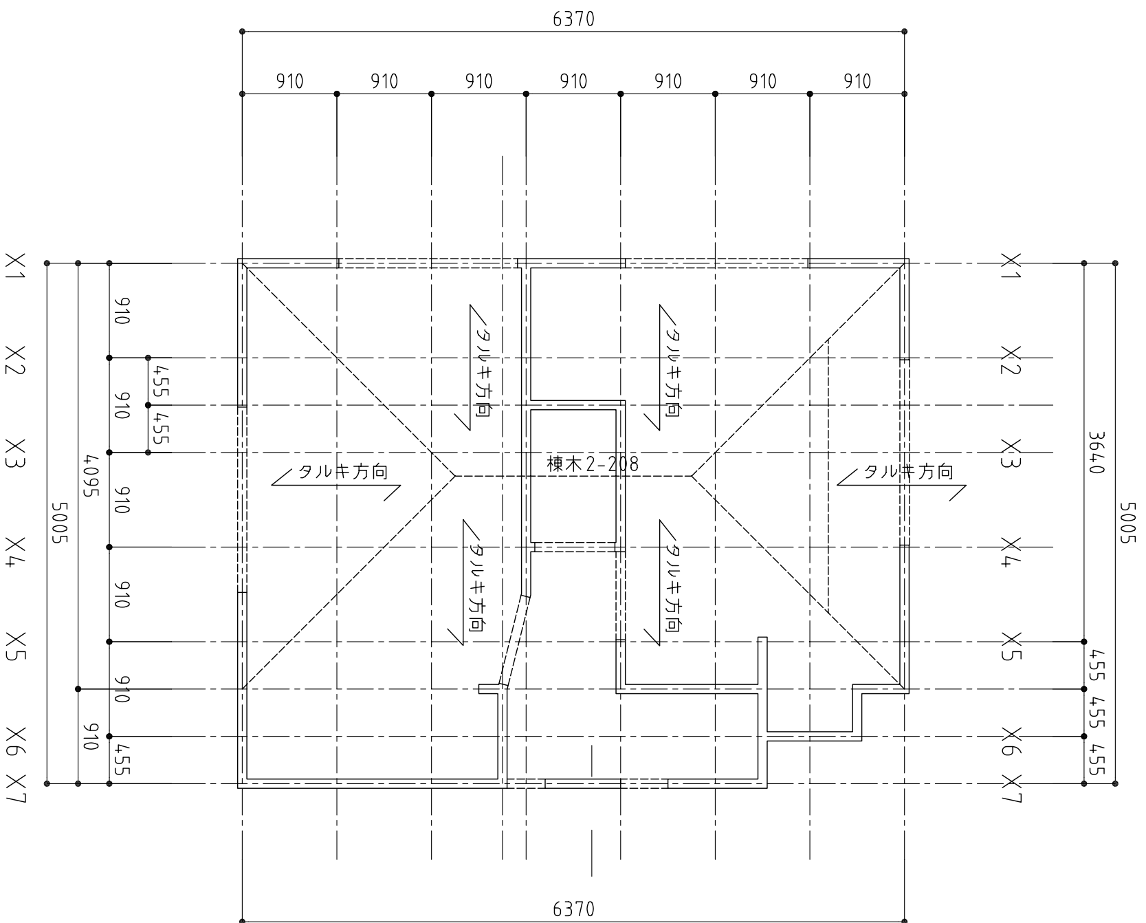
棟木・タルキ方向伏図 S=1/50
