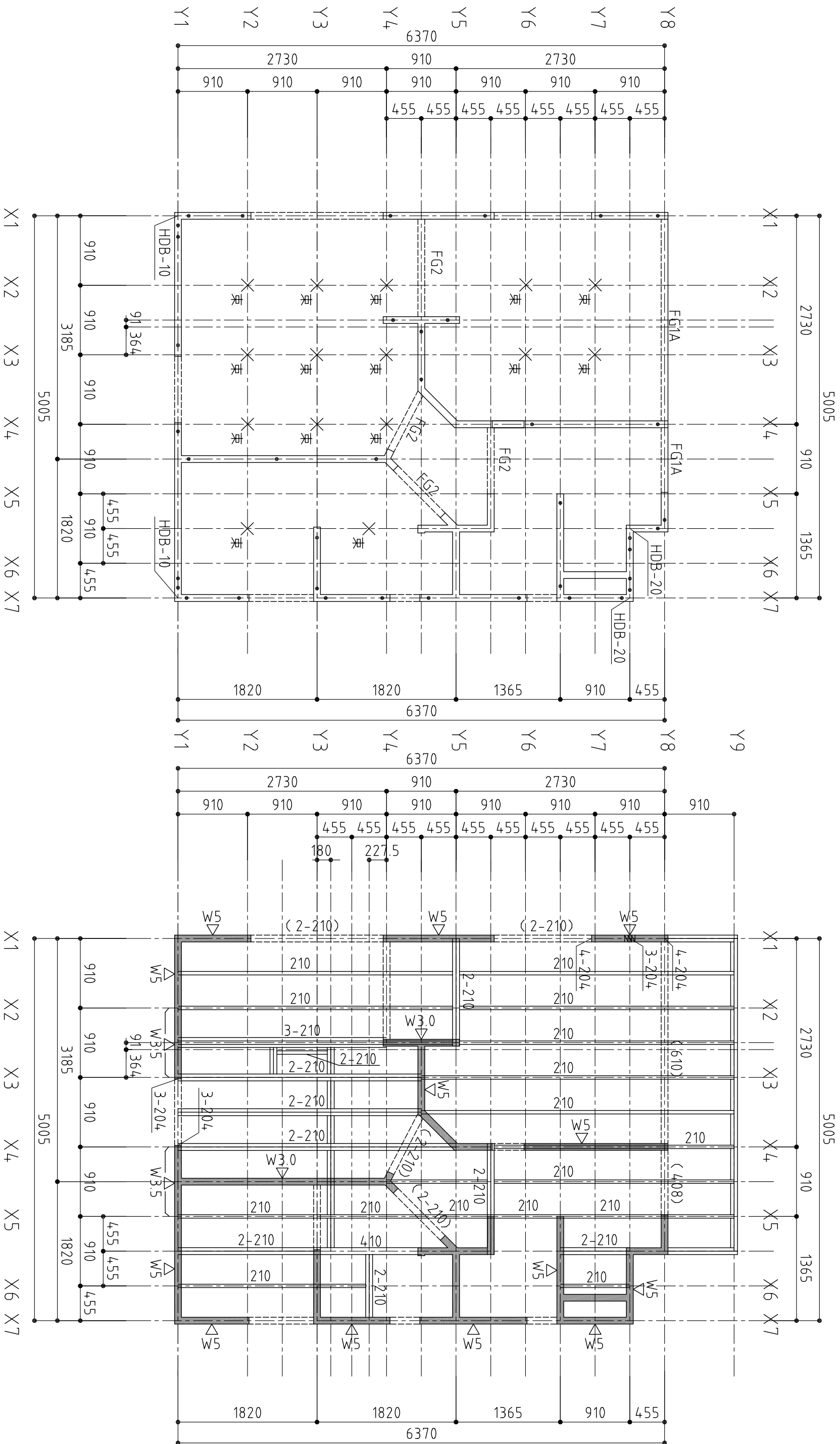
基礎伏図 S=1/50
